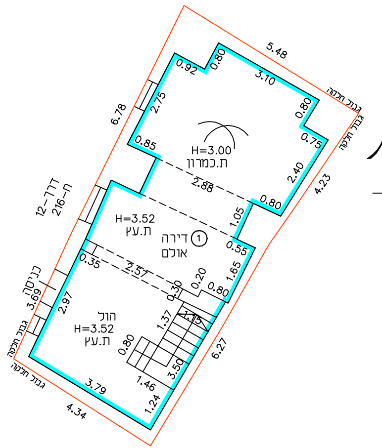
תכנית קומה קרקע קנ"מ 1:100
