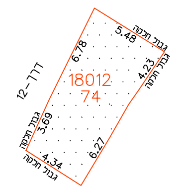
תרשים החלקה קנ"מ 1:250
