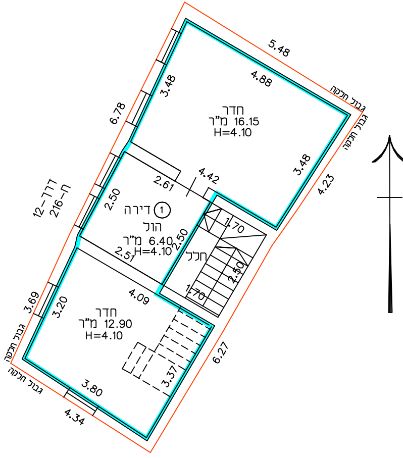
תכנית קומה ראשונה קנ"מ 1:100
